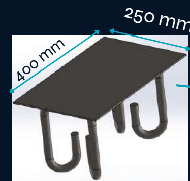
Anclajes tipo A
